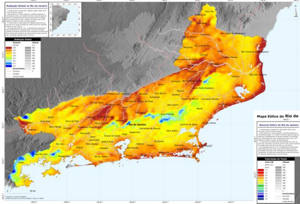
Mapa de Radiação Solar do Rio de Janeiro, Brasil
