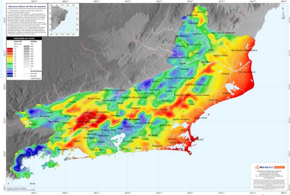
Mapa Eólico do Rio de Janeiro, Brasil
